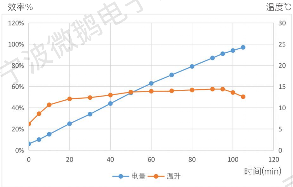
三星S7充电过程温升曲线
